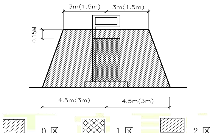
图 3.9-2 汽油加油机爆炸危险区域划分
