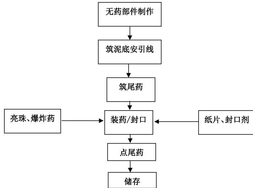
图 2-4-3 效果内筒生产流程图
