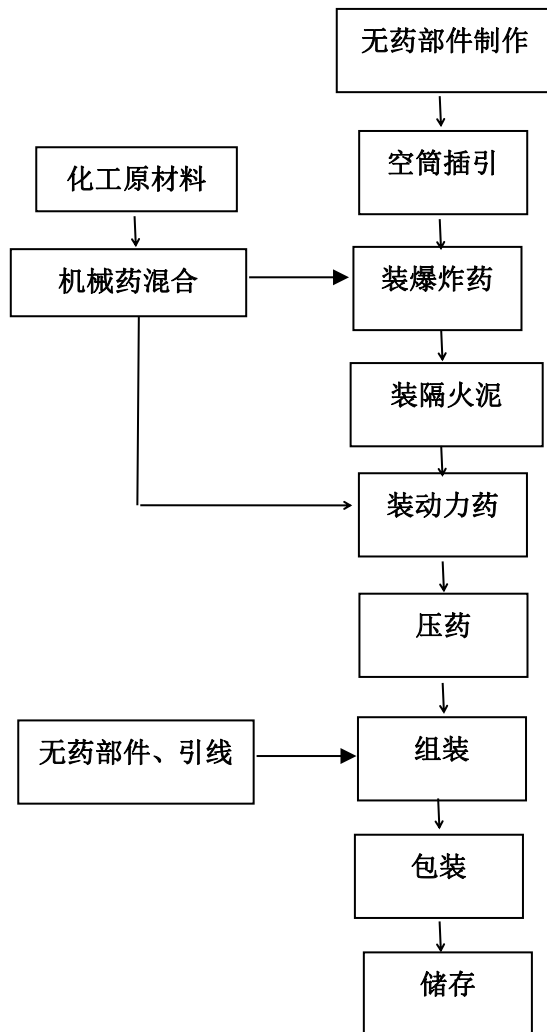
图 2-4-5 升空类（双响炮）生产流程图
