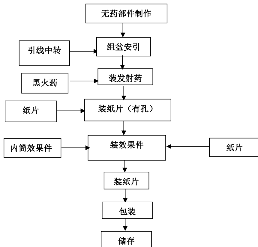
图 2-4-4 组合烟花产品生产工艺流程图
