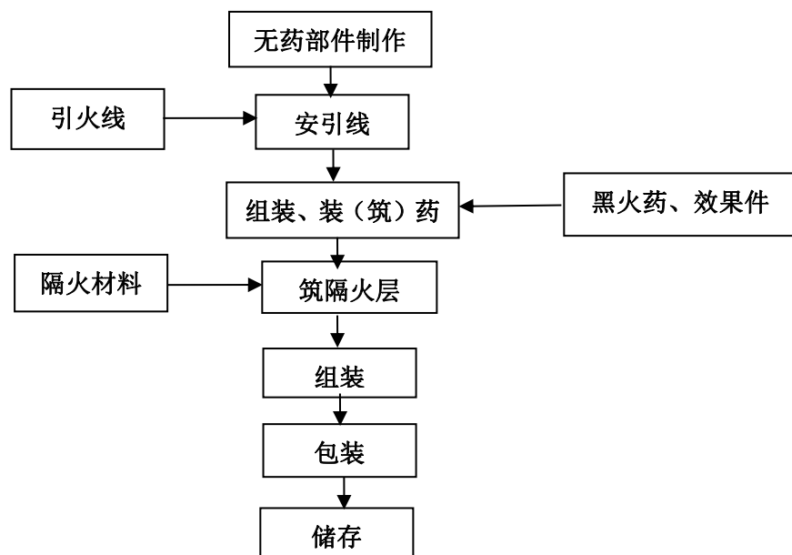
图 2-4-1 吐珠类产品生产工艺流程图
